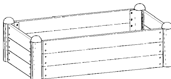
140 × 80 cm, 36 cm hoch
