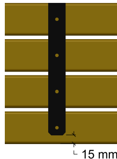
Bankmitte mit Mittelstrebe B (Kreis in der Mitte)
